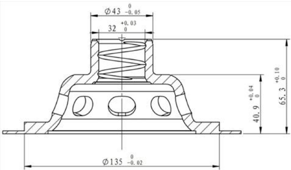
被测工件尺寸图
